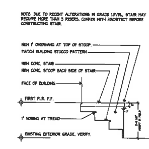
14 SECTION THRU NEW EXTERIOR STA A8.3 SCALE: 1/2"=1'-0"
